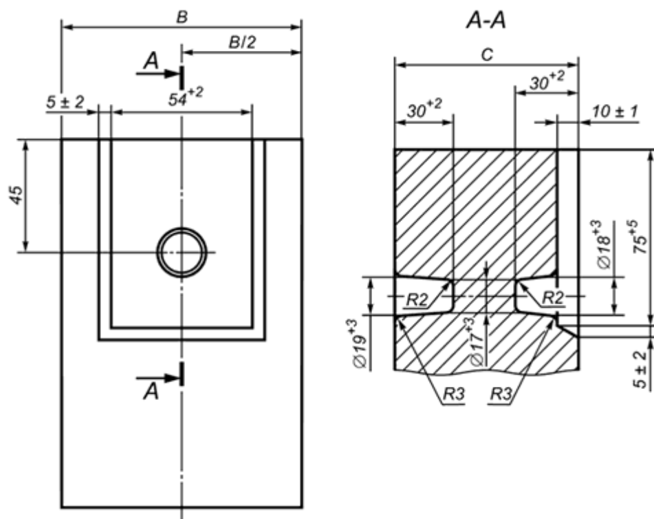
Рисунок А.7 - Размеры углублений для подвески. Вариант 2
