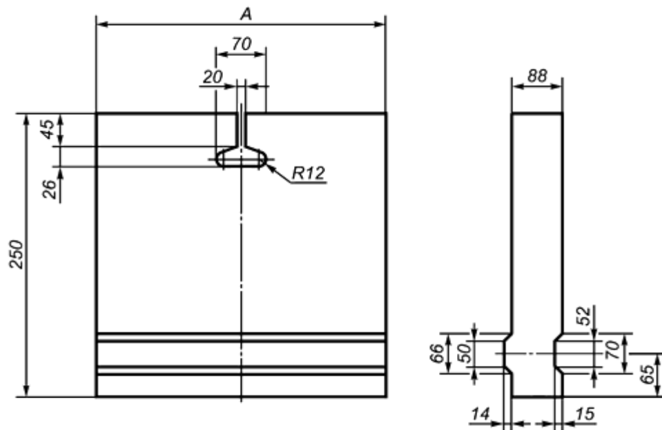
Рисунок 14 - Сводные фасонные изделия 84, 85
