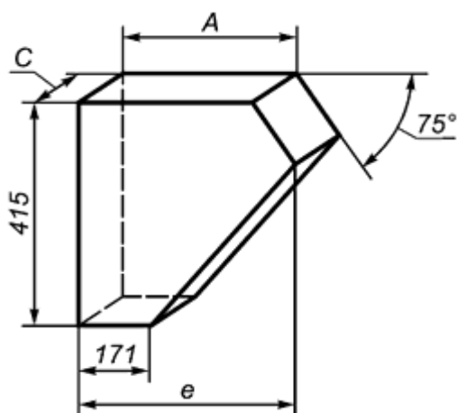
Рисунок 26 - Насадочные фасонные изделия 130-135
