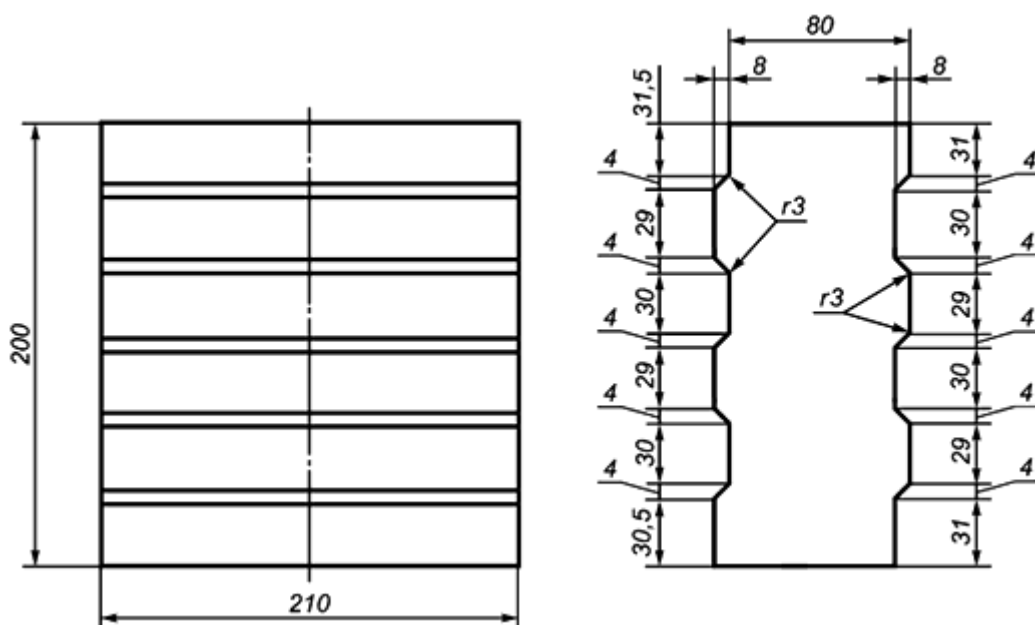
Рисунок 24 - Сводовое фасонное изделие 118
