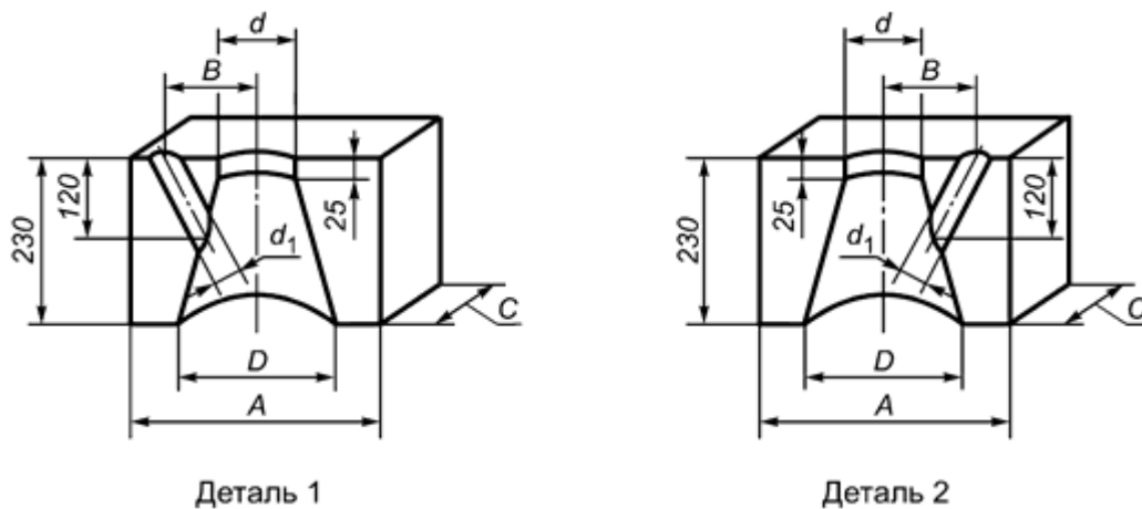
Рисунок 36 - Горелочные фасонные изделия 98-102
