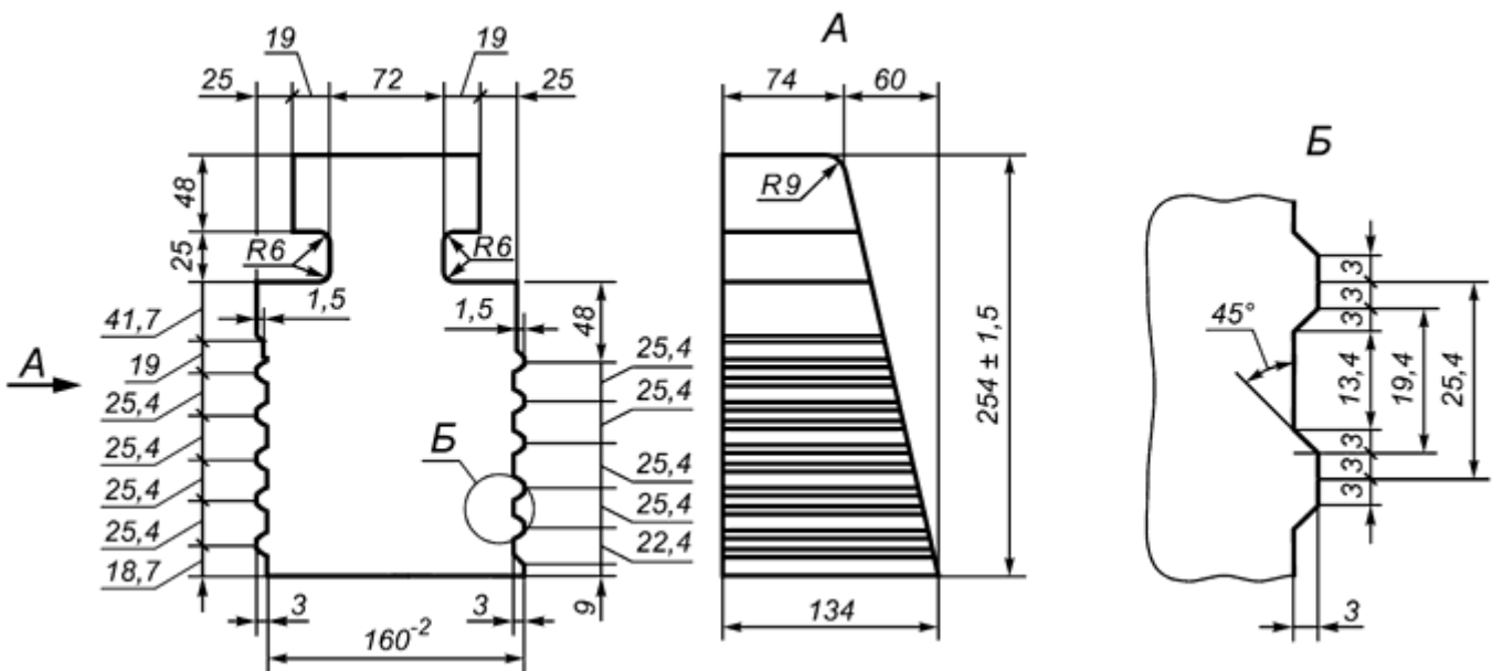
Рисунок 10 - Сводное фасонное изделие 79
