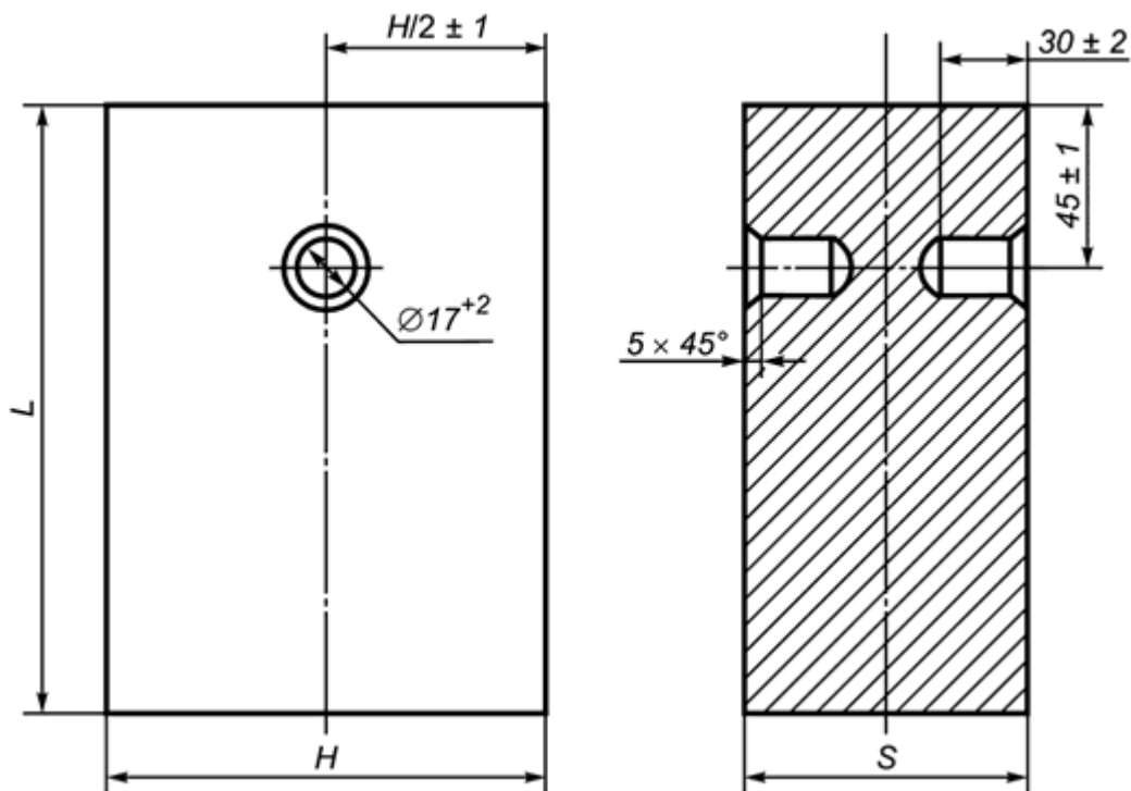
Рисунок А.1 - Размеры отверстий для штырей. Вариант 1
