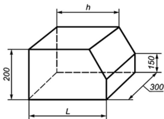
Рисунок 41 - Фасонные изделия 169, 170 (фасонный брусок)
