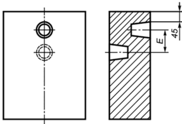
Рисунок А.2 - Размеры отверстий для штырей. Вариант 2
