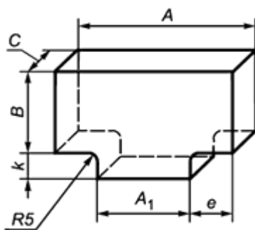
Рисунок 25 - Насадочные фасонные изделия 119-129
