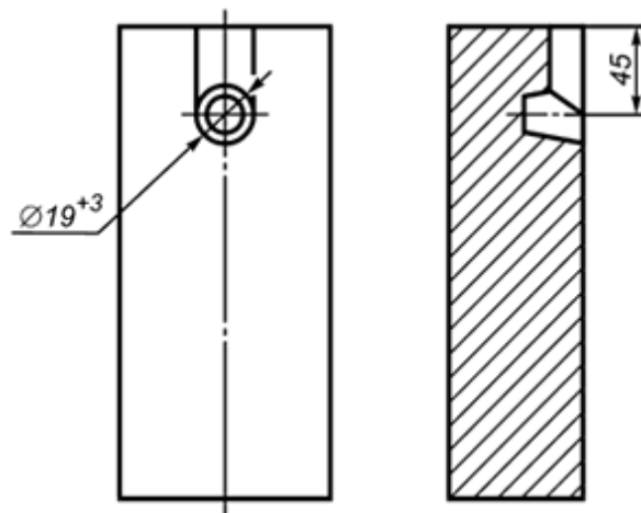
Рисунок А.9 - Размеры углублений для подвески. Вариант 4
