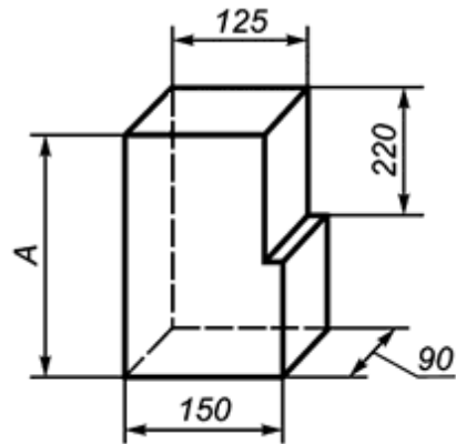
Рисунок 37 - Опорные фасонные изделия 163-165
