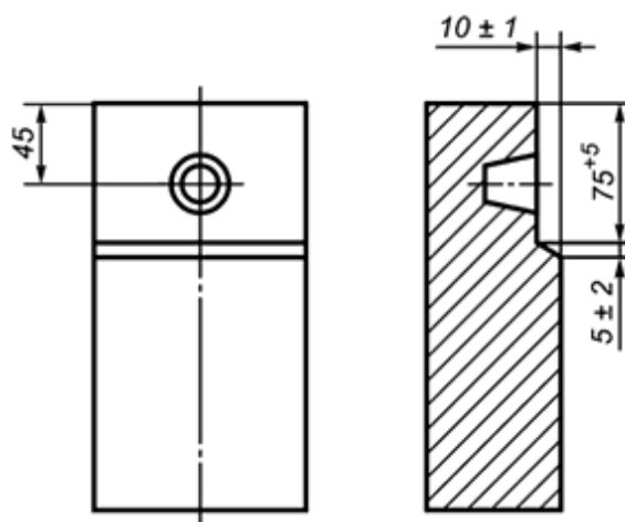
Рисунок А.9 - Размеры углублений для подвески. Вариант 4
