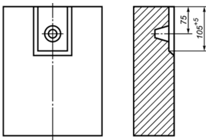
Рисунок А.7 - Размеры углублений для подвески. Вариант 2
