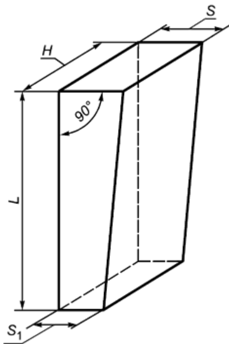
а - Односторонний полуторный торцовый клин
