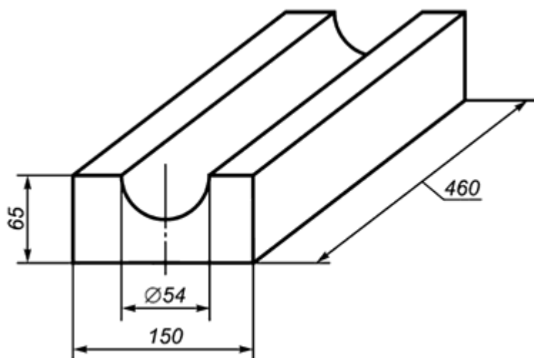
Рисунок 39 - Фасонное изделие с контрольным отверстием 167
