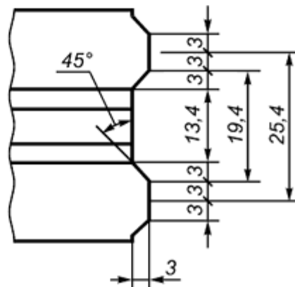
Рисунок 9 - Сводные фасонные изделия 76-78 Таблица 9 - Сводные фасонные изделия 76-78
