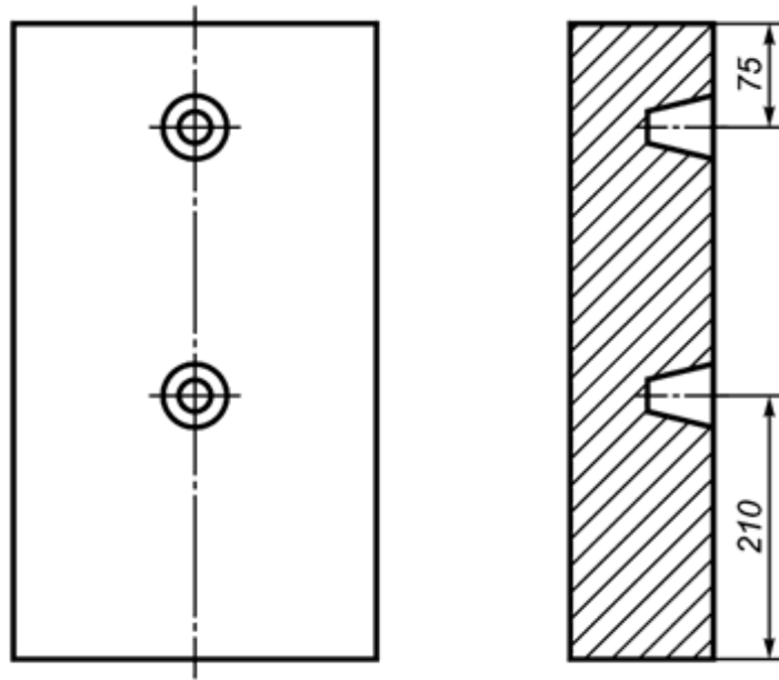
Рисунок А.4 - Размеры отверстий для штырей. Вариант 4
