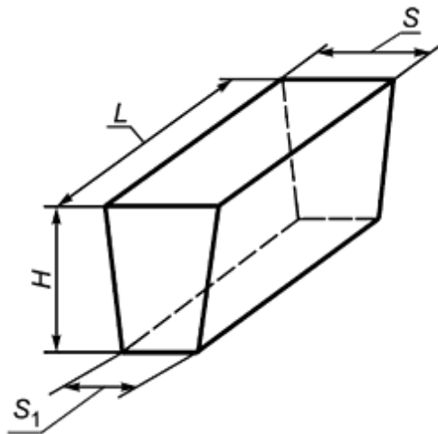
а - Односторонний ребровой клин
