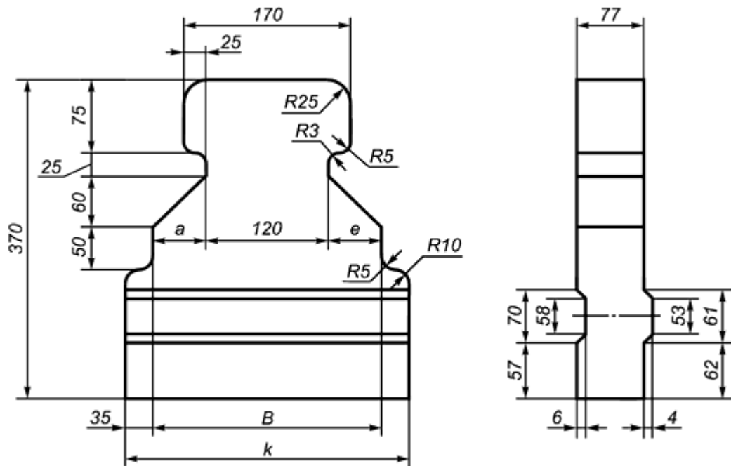
Рисунок 17 - Сводные фасонные изделия 88-90
