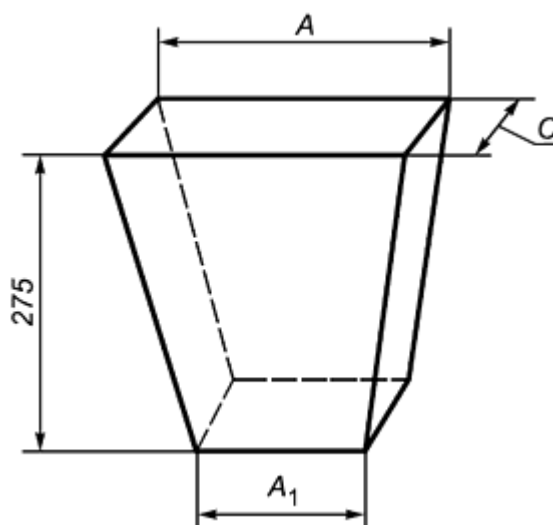
Рисунок 27 - Насадочные фасонные изделия 136-141
