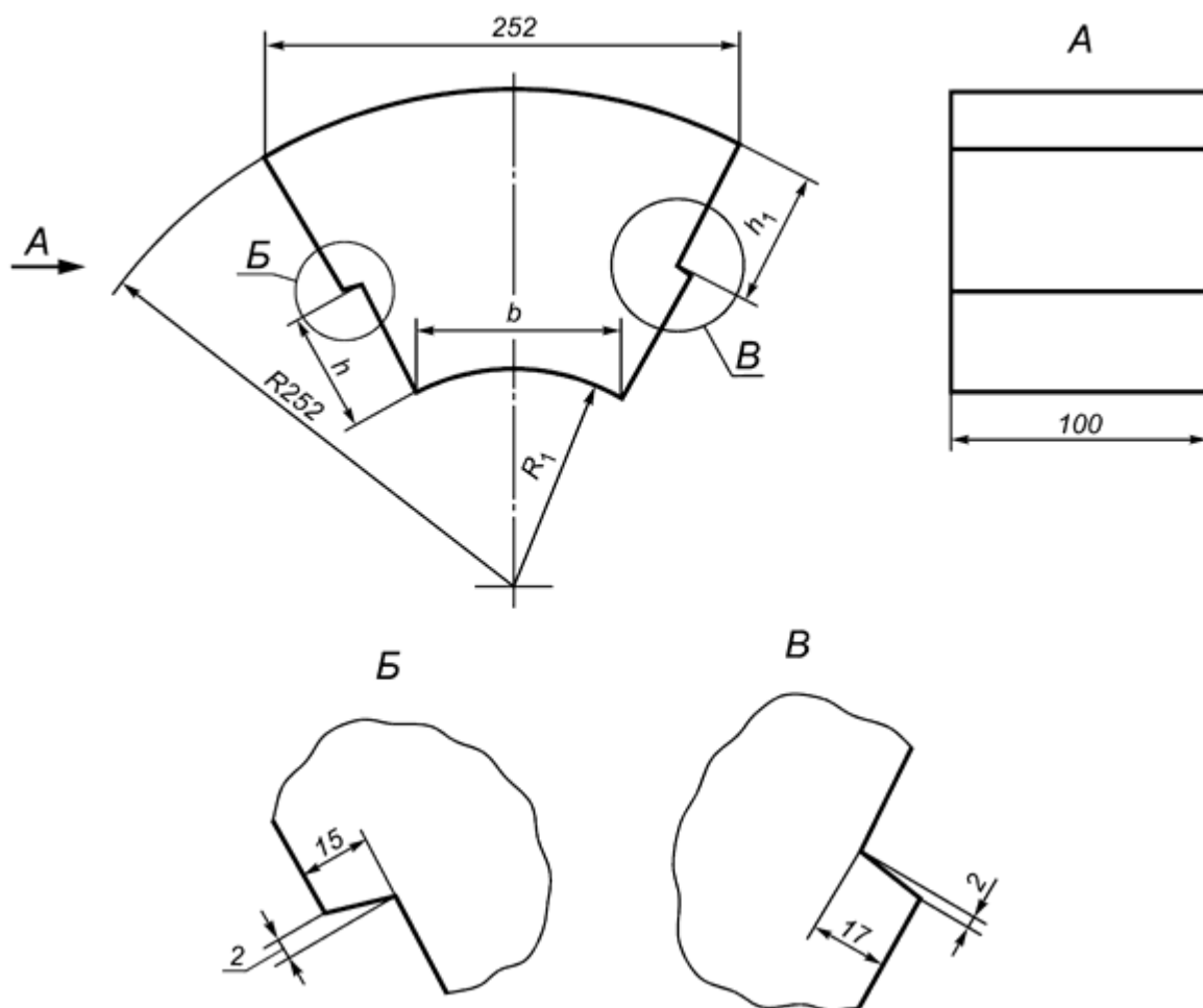
Рисунок 31 - Секторные фасонные изделия 144, 145
