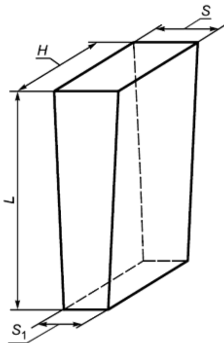
б - Двухсторонний полуторный торцовый клин Рисунок 3 - Полуторные торцовые клины
