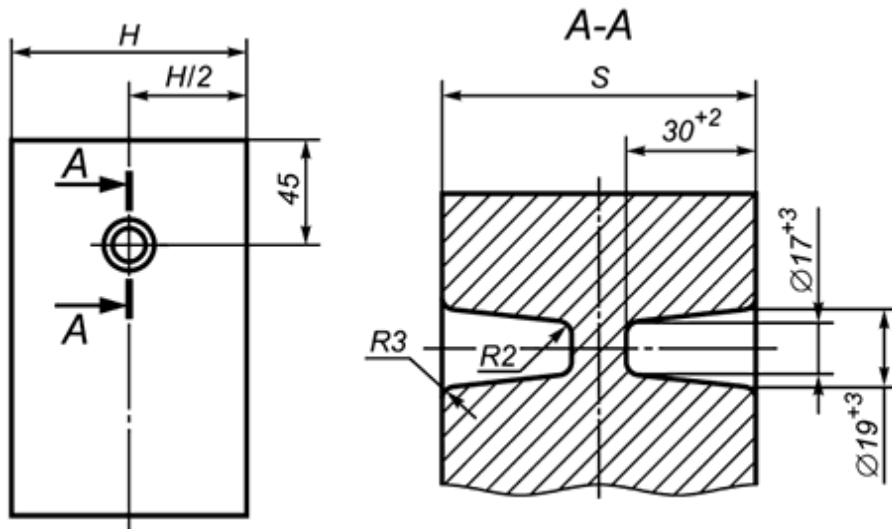
Рисунок А.2 - Размеры отверстий для штырей. Вариант 2
