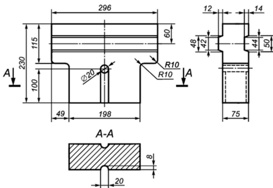
Рисунок 18 - Сводное фасонное изделие 91
