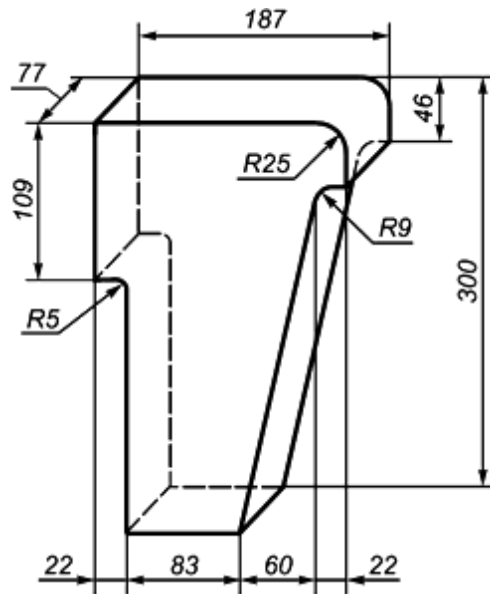
Рисунок 12 - Сводовое фасонное изделие 81
