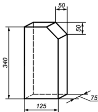
Рисунок 39 - Фасонное изделие с контрольным отверстием 167
