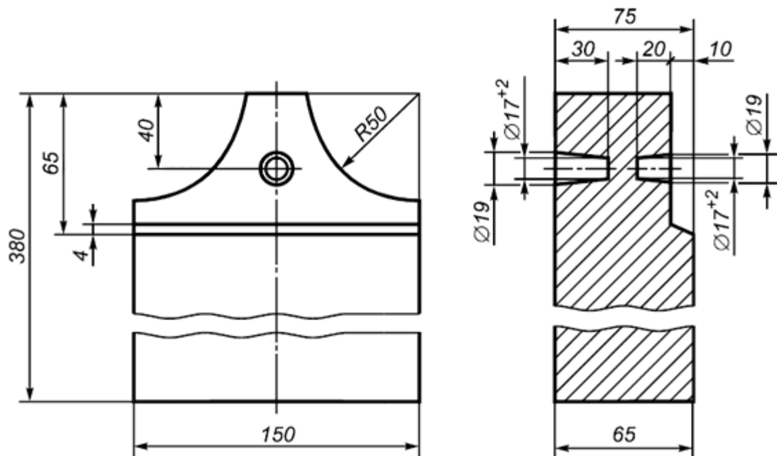
Рисунок 22 - Сводное фасонное изделие 114
