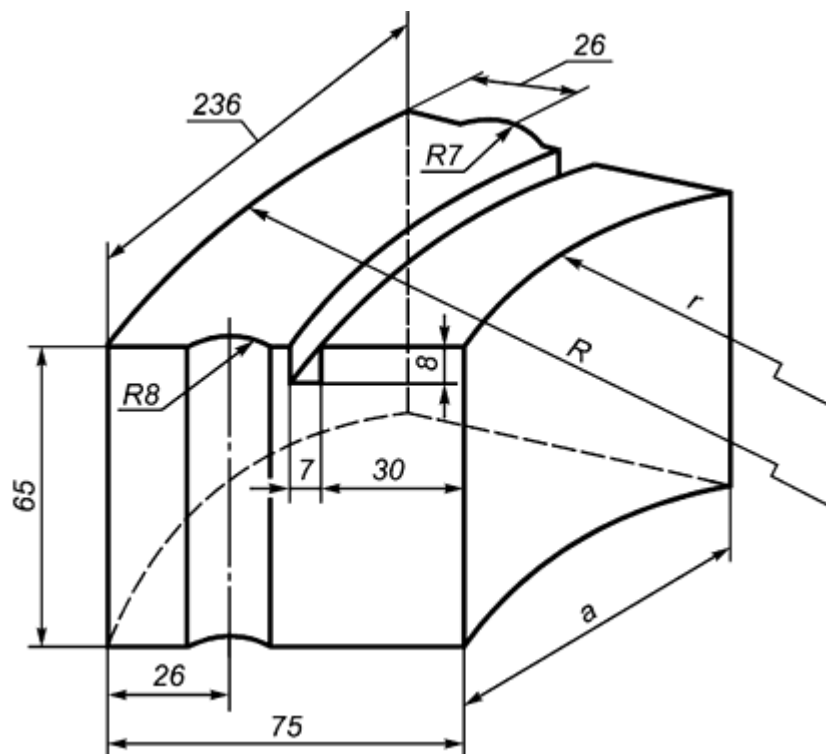
Рисунок 28 - Секторные фасонные изделия 103-109
