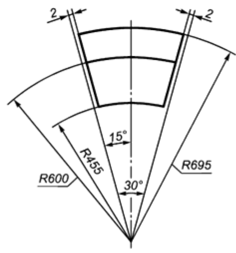
Рисунок 29 - Секторное фасонное изделие 142
