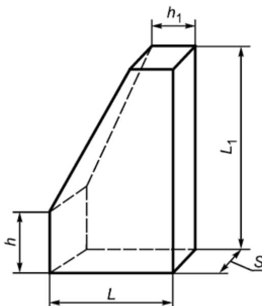
Рисунок 8 - Оконный пятовый кирпич
