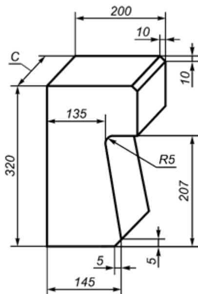
Рисунок 35 - Бортовые фасонные изделия 92, 93
