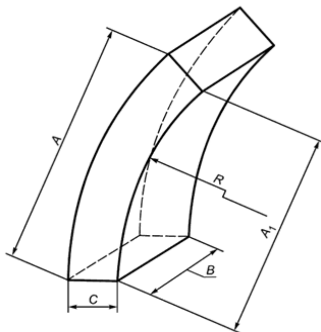
Рисунок 33 - Секторные фасонные изделия 148-150
