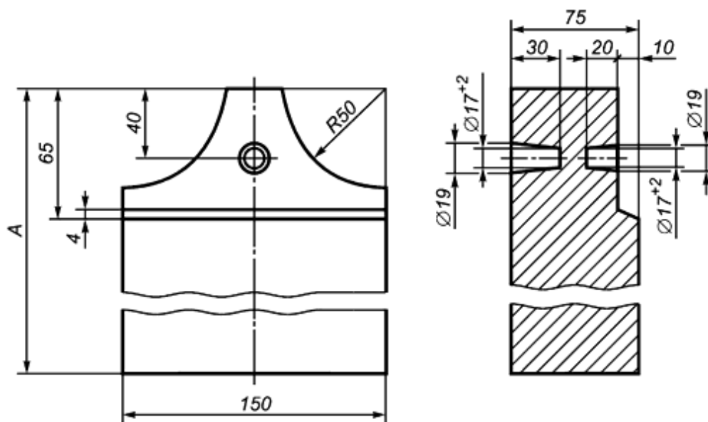
Рисунок 21 - Сводовые фасонные изделия 112, 113
