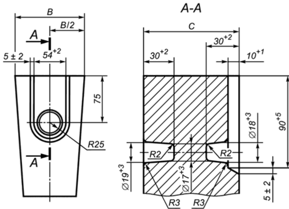
Рисунок А.6 - Размеры углублений для подвески. Вариант 1
