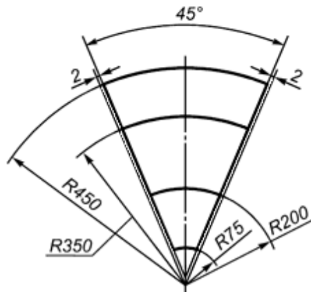
Рисунок 30 - Секторное фасонное изделие 143
