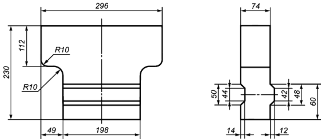
Рисунок 15 - Сводное фасонное изделие 86
