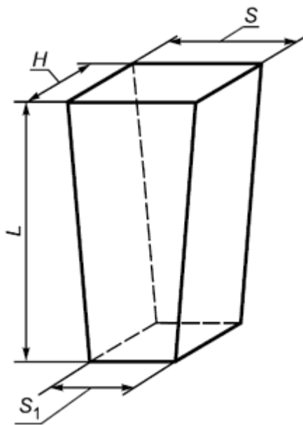
а - Односторонний трапецидальный клин
