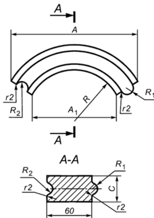
Рисунок 34 - Секторные фасонные изделия 151-162
