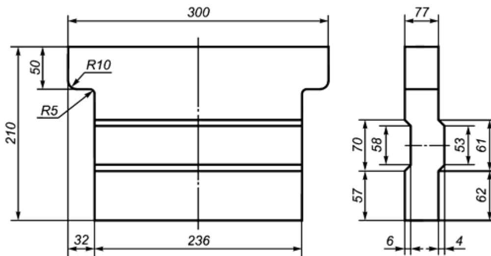
Рисунок 18 - Сводное фасонное изделие 91
