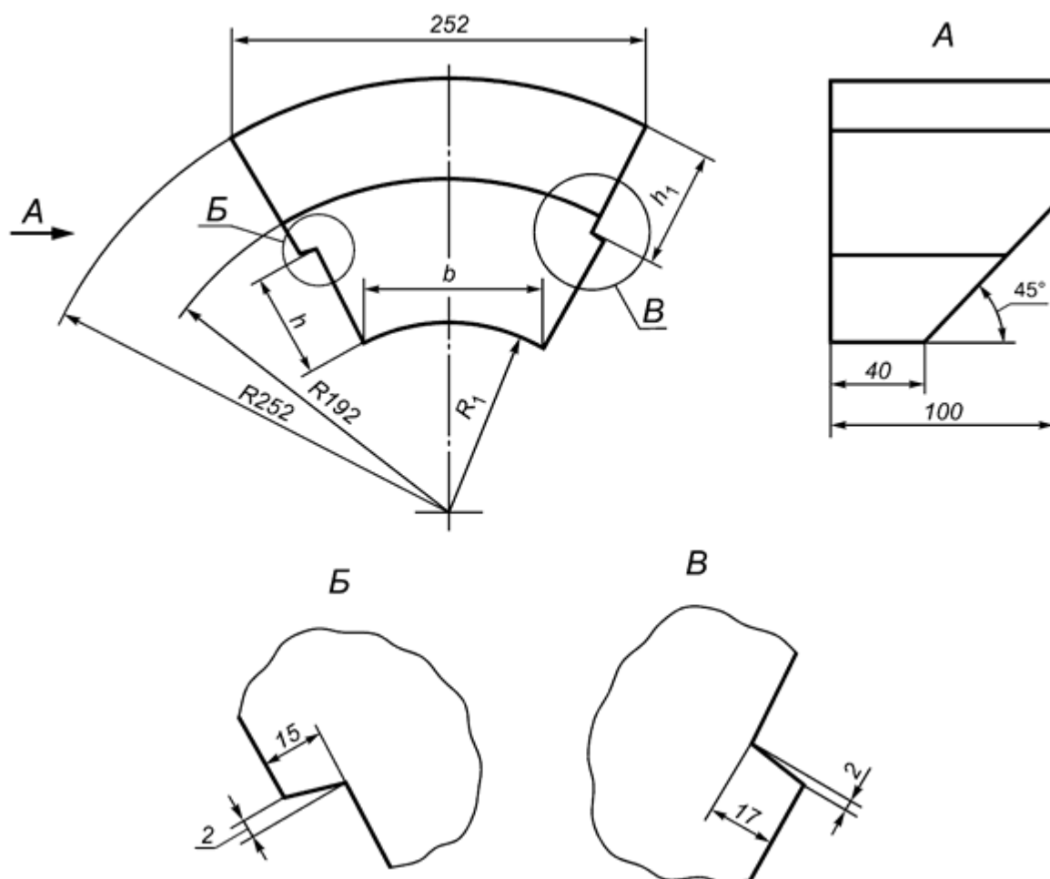
Рисунок 32 - Секторные фасонные изделия 146, 147
