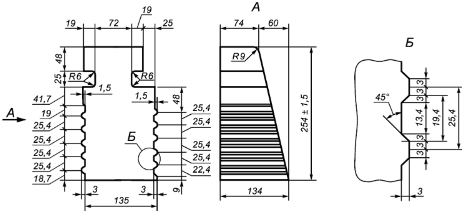
Рисунок 10 - Сводное фасонное изделие 79
