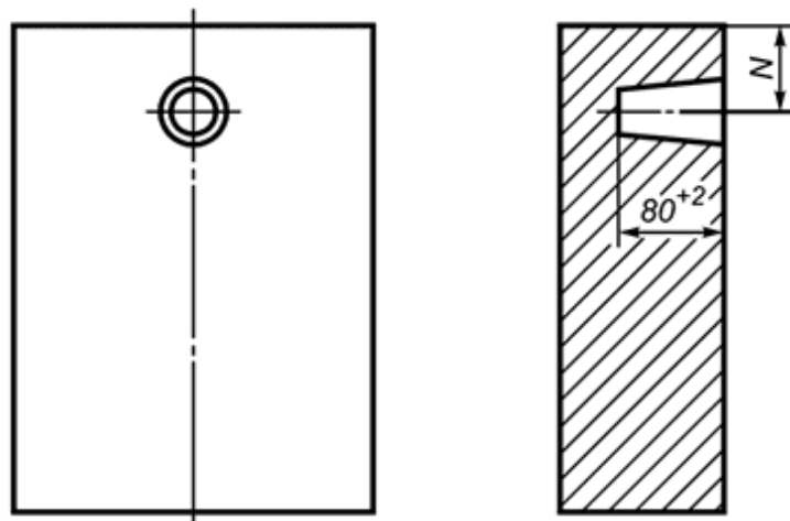
Рисунок А.3 - Размеры отверстий для штырей. Вариант 3
