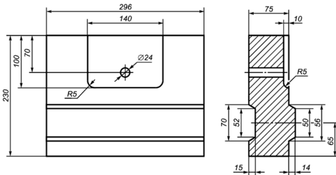
Рисунок 20 - Сводовое фасонное изделие 111
